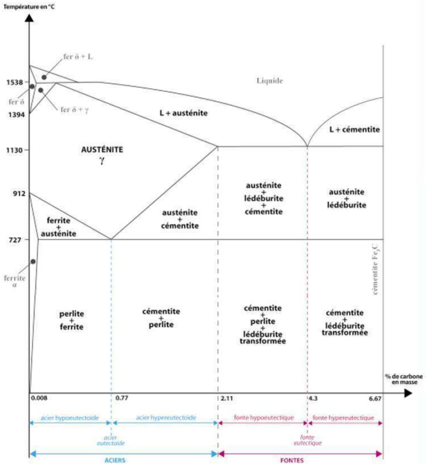
Diagramme de phase fer/carbone
